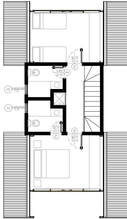
PLANTA ALTA
